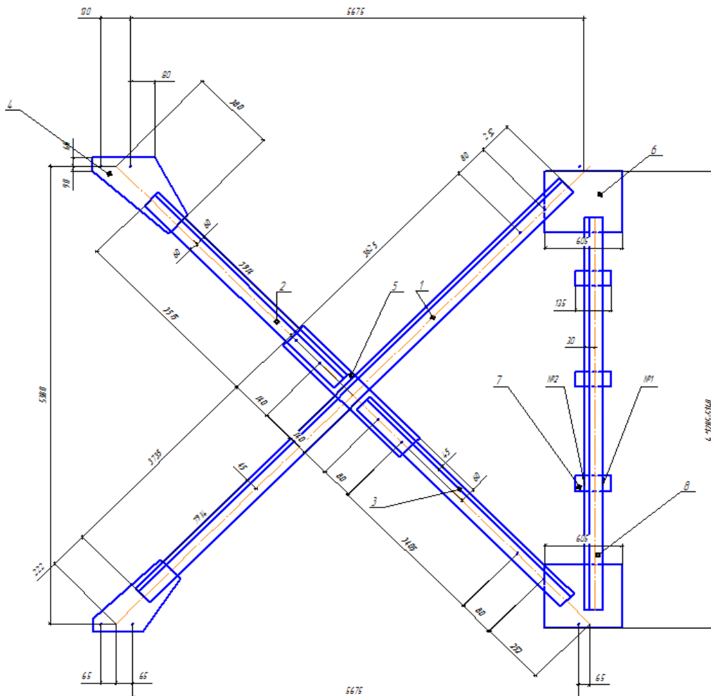
Рисунок 2.1 – Эскиз сварной конструкции
