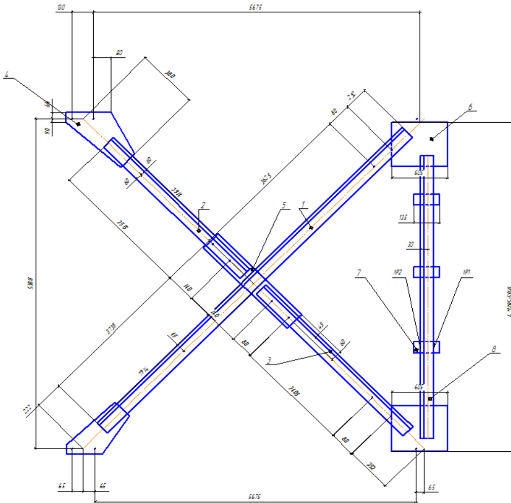
Рисунок 2.1 – Эскиз сварной конструкции
