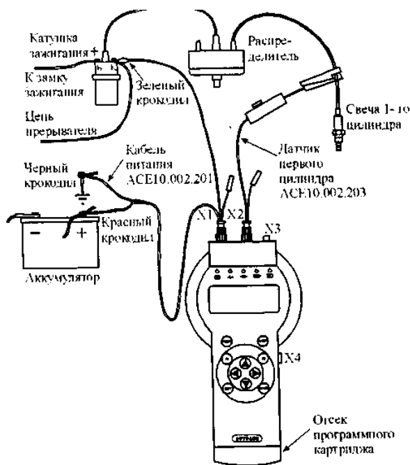
Рис.6. Схема подключения прибора к автомобилю с механическим распределителем высоковольтной энергии
