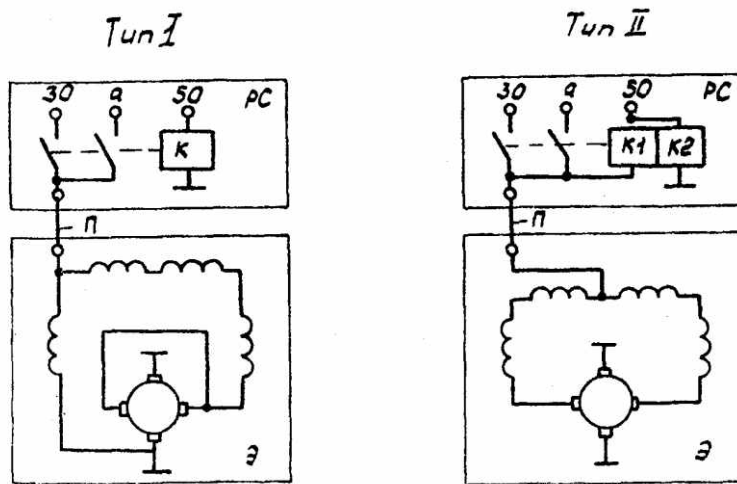
Рис.5. Основные типы электрических схем стартеров: РС – тяговое реле стартера; Э – электродвигатель стартера; К – обмотка реле; К1 – втягивающая обмотка; К2 – удерживающая обмотка; П – переключатель; 30 – к аккумуляторной батарее; 50 – к реле включения стартера
