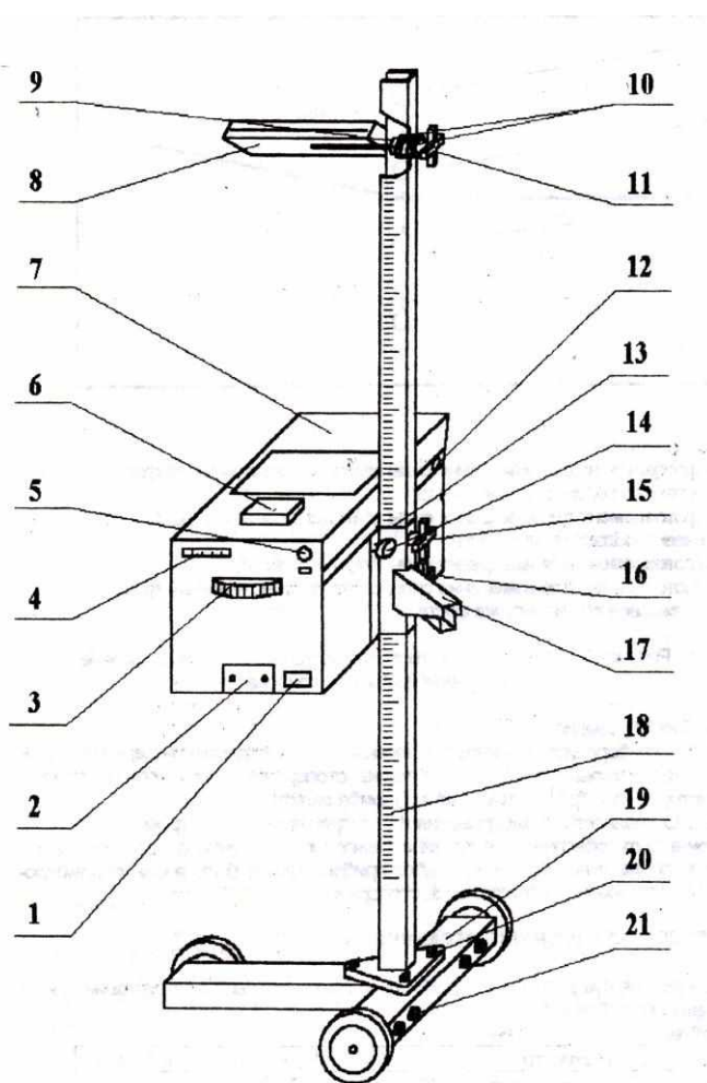
Рисунок 1 - Прибор для проверки и регулировки света фар модели ОП.
