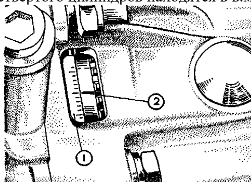
Рис. 2. Метки для установки момента зажигания: 1 - шкала; 2 - метка на маховике
