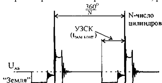
Рис.22. Угол замкнутого состояния контактов
