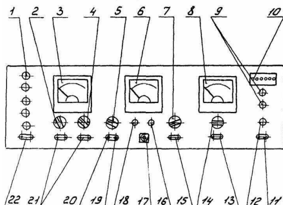
Рис.2. Панель приборов
