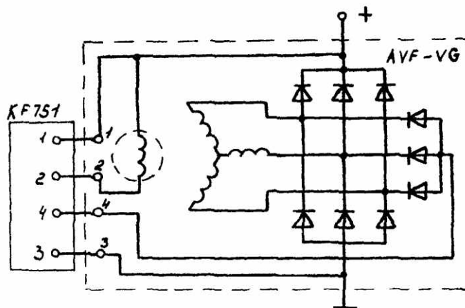
Рис.10. Схема генератора с обмоткой возбуждения, запитываемой от отдельного выпрямителя
