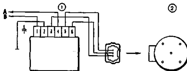
Рис. 4. Схема для снятия характеристик датчика-распределителя зажигания на стенде: 1 - коммутатор; 2 - датчик-распределитель зажигания; А - к клемме "+" стенда; В - к клемме "прерыватель" стенда
