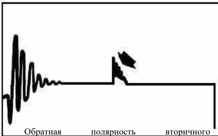
Рис. 12. Осциллограмма вторичного напряжения. Нормальное изображение
