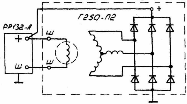
Рис.4. Схема генератора с обмоткой возбуждения и с двумя изолированными выводами
