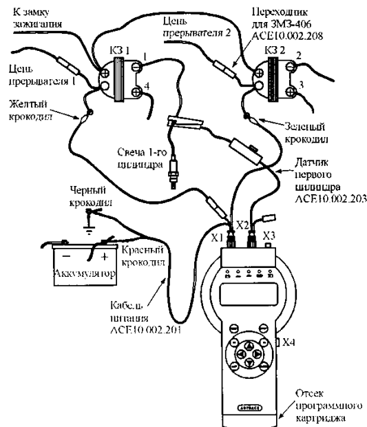
Рис.12. Схема подключения прибора к автомобилю со статическим распределением высоковольтной энергии с двумя двухвыводными катушками зажигания (на примере автомобиля «Волга» с двигателем ЗМЗ-406)
