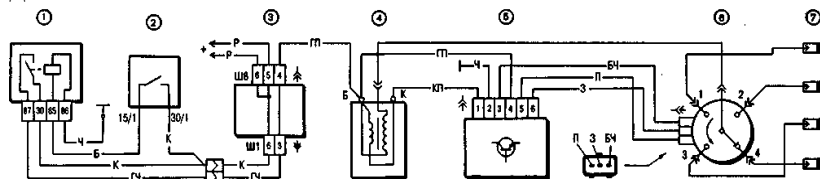
Рис. 1. Схема системы зажигания: 1 - реле зажигания; 2 - выключатель зажигания; 3 - монтажный блок; 4 - катушка зажигания; 5 - коммутатор; 6 - датчик-распределитель зажигания; 7 - свечи зажигания
