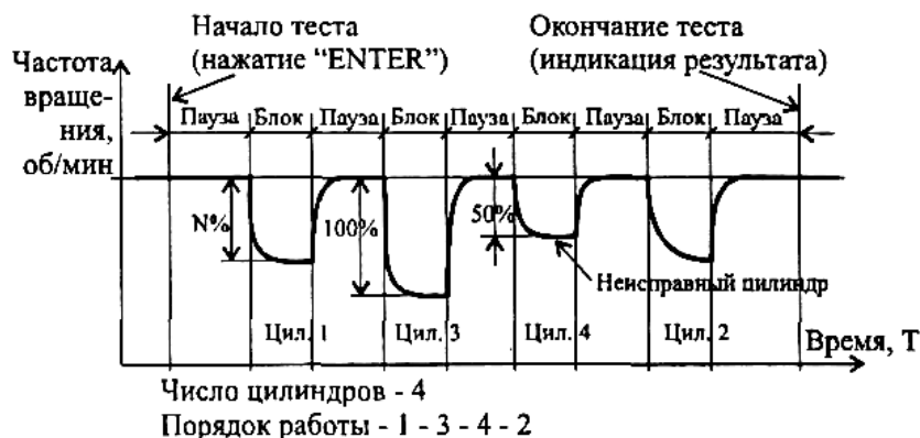
Рис.15. Баланс мощности четырехцилиндрового двигателя
