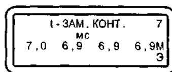
Рис.28. Тест «t-замыкания контактов»
