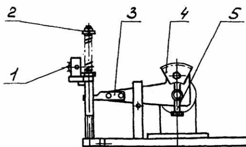
Рис.4. Тормоз
