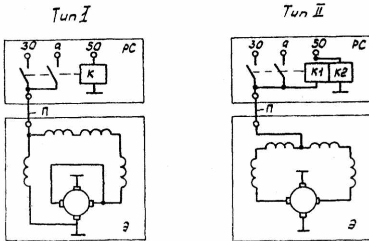
Рис.5. Основные типы электрических схем стартеров: РС – тяговое реле стартера; Э – электродвигатель стартера; К – обмотка реле; К1 – втягивающая обмотка; К2 – удерживающая обмотка; П – перемычка; 30 – к аккумуляторной батарее; 50 – к реле включения стартера
