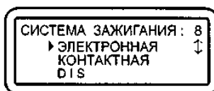
Рис.8. Меню выбора системы зажигания
