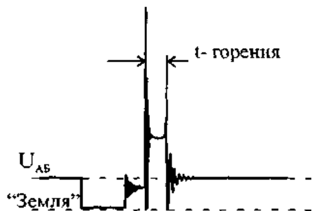
Рис.29. t-горения
