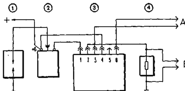
Рис. 9. Схема для проверки коммутатора: 1 - разрядник; 2 - катушка зажигания; 3 - коммутатор; 4 - резистор 0,01 \text{ Ом} \pm 1 \% , 220 Вт; А - к генератору прямоугольных импульсов В - к осциллографу
