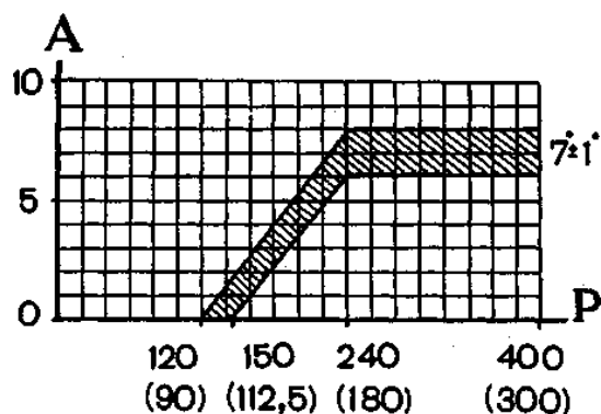
Рис. 6. Характеристика вакуумного регулятора датчика-распределителя зажигания: А - угол опережения зажигания, град; Р - разрежение, гПа (мм рт. ст.)
