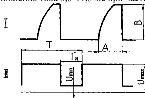
Рис. 10. Форма импульсов на экране осциллографа: I - импульсы коммутатора; II - импульсы генератора; А - время накопления тока; В - максимальная величина тока
