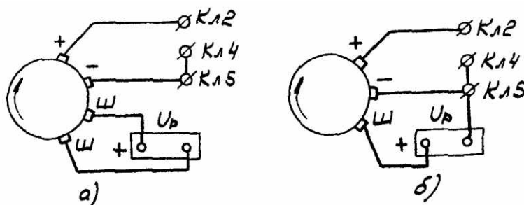
Рис.11. Схема подключения генераторов переменного тока при проверке в режиме холостого хода и под нагрузкой: а – с обмоткой возбуждения
