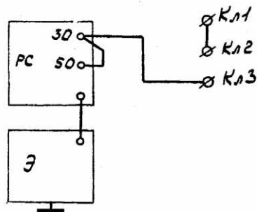
Рис.6. Схема включения стартера при проверке в режиме холостого хода
