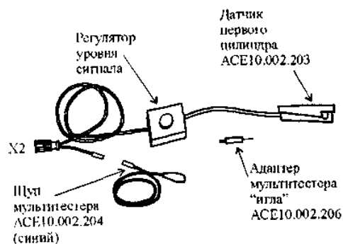
Рис.10. Датчик первого цилиндра (ACE10.002.203)
