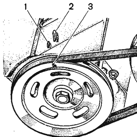
Рис. 3. Метки для установки момента зажигания: 1 - метка опережения зажигания на 5^\circ ; 2 - метка опережения зажигания на 0^\circ ; 3 - метка в.м.т. на шкиве коленчатого вала
