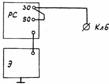
Рис.8. Схема включения стартера при проверках в режиме холостого хода и полного торможения
