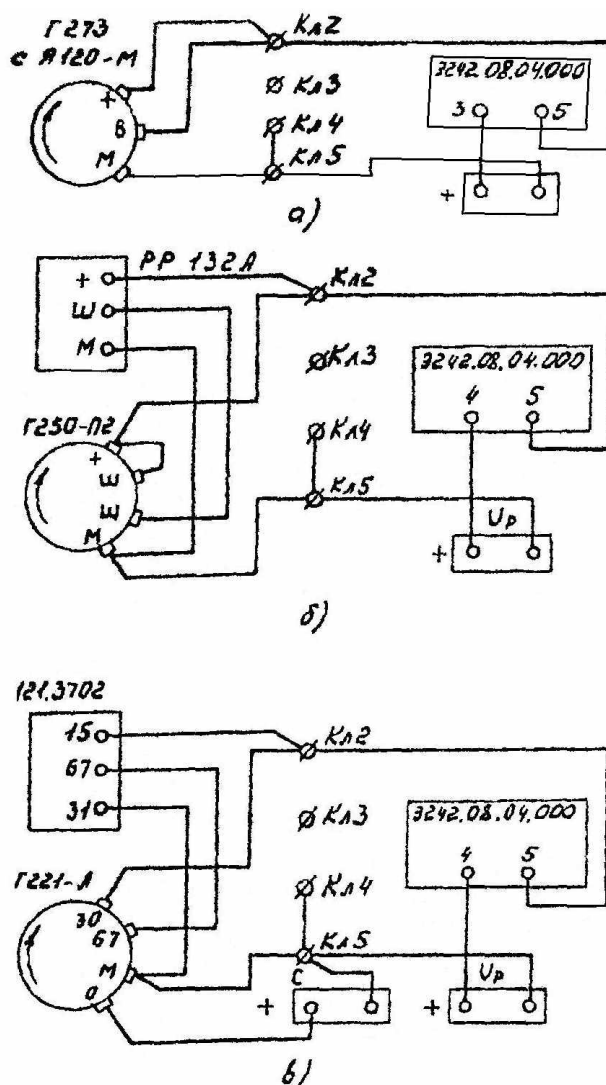
Рис.5. Схемы подключения генераторных установок при проверке регуляторов напряжения
