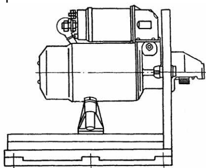
Рис.3. Установка стартера в нагрузочном устройстве
