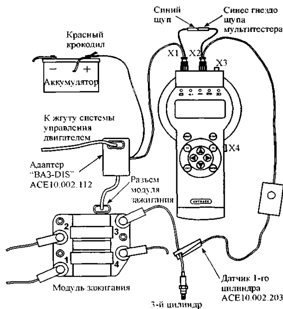
Рис.15. Схема подключения прибора к автомобилю со статическим распределением высоковольтной энергии (DIS) с модулем зажигания (на примере автомобилей «ВАЗ» с двигателями 2111, 2112)
