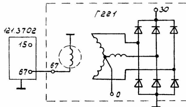
Рис.5. Схема генератора с обмоткой возбуждения, соединенной одним выводом с корпусом генератора: 15 – к «+» бортовой сети через выключатель зажигания; 67 – к корпусу генератора; 30 – к потребителям; 0 – к выводу реле контрольной лампы
