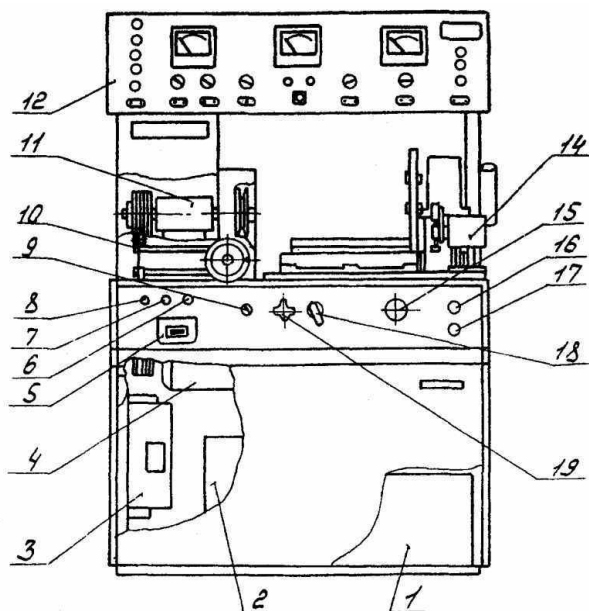
Рис.1. Стенд контрольно-испытательный
