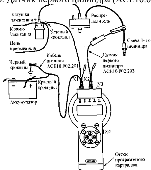
Рис.10. Датчик первого цилиндра (ACE10.002.203)
