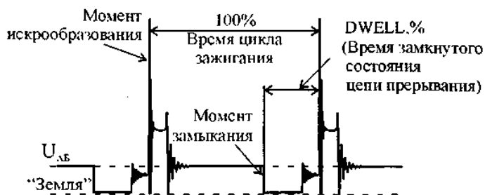
Рис.26. DWELL
