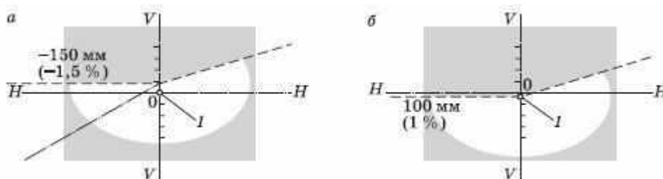
Рис. Установка фотоприемника при измерении силы света фар ближнего света: а — в освещенной части измерительного экрана; б — в теневой части измерительного экрана; I — фотоприемник
