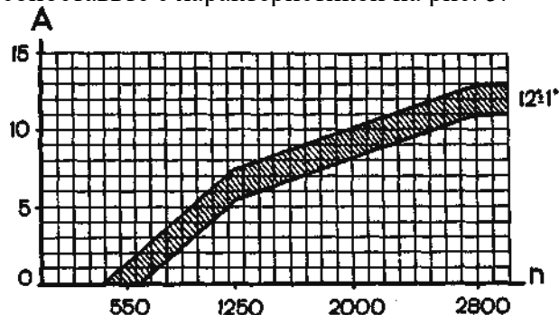
Рис. 5. Характеристика центробежного регулятора датчика-распределителя зажигания: А - угол опережения зажигания, град; n - частота вращения валика датчика-распределителя зажигания, мин-1
