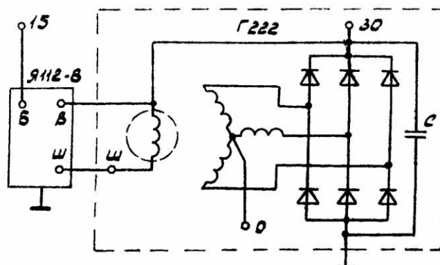
Рис.9. Схема генератора с обмоткой возбуждения, соединенной одним выводом с выходом генератора: 15 – к выводу «+» аккумуляторной батареи; 30 – к потребителям; 0 – к выводу реле контрольной лампы
