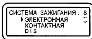
Рисунок 8 - Меню выбора системы зажигания
