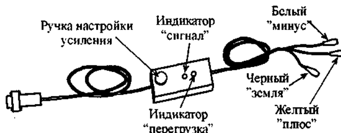
Рисунок 10 - Адаптер электронный «УОЗ» (АСЕ10.002.106)
