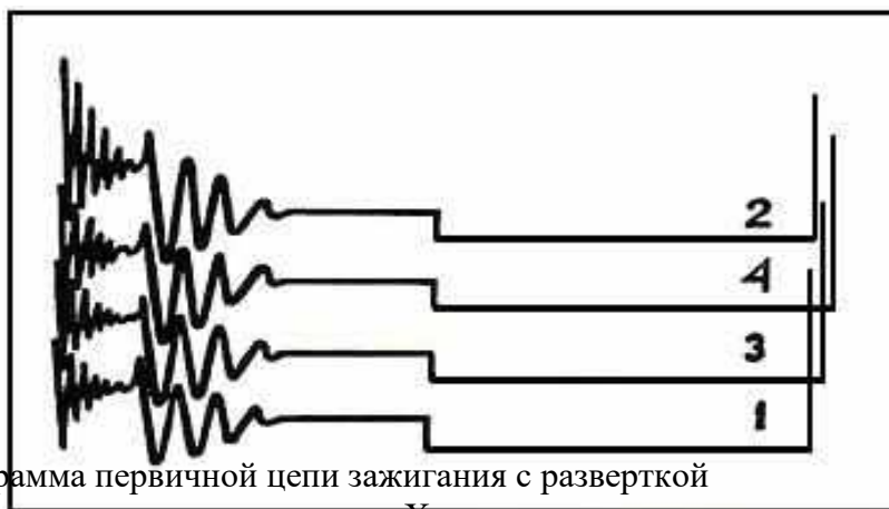
Рис. 6. Зоны, характеризующие неисправности катушки зажигания и конденсатора
