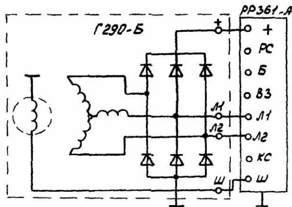
Рис.6. Схема генератора с дополнительными фазными выводами
