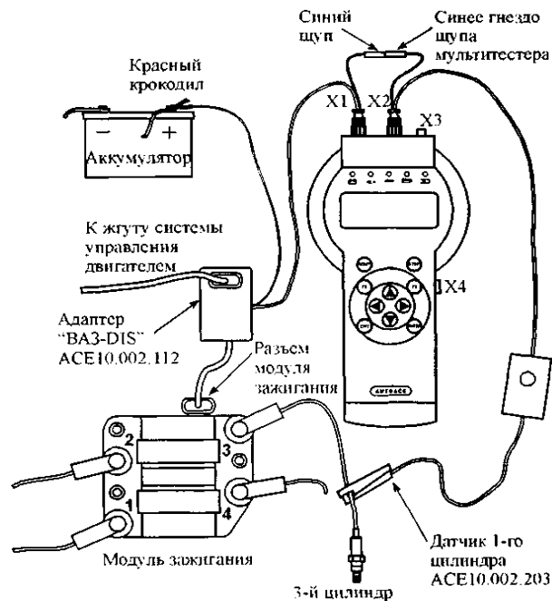
Рис.8. Схема подключения прибора к автомобилю со статическим распределением высоковольтной энергии (DIS) с модулем зажигания (на примере автомобилей «ВАЗ» с двигателями 2111, 2112)
