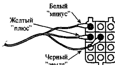
Рисунок 11 - Пример подключения прибора при выполнении теста «УОЗ» к колодке диагностики ВМТ ВАЗ
