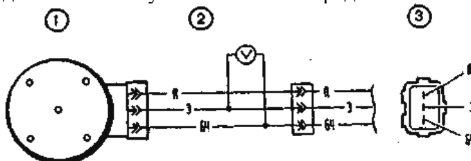
Рис. 8. Схема для проверки бесконтактного датчика на автомобиле: 1 - датчик-распределитель зажигания; 2 - переходный разъем с вольтметром, имеющим предел шкалы не менее 15 В и внутреннее сопротивление не менее 100кОм; 3 - вид на штепсельный разъем датчика-распределителя зажигания
