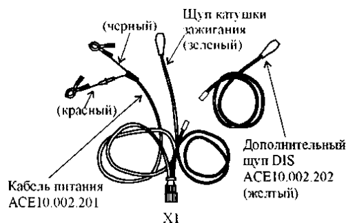
Рис.9. Кабель питания ACE10.002.201
