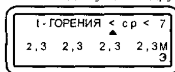
Рис.30. Тест «t-горения»
