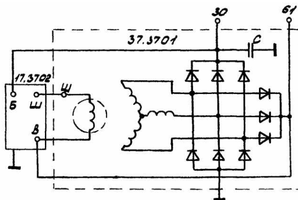
Рис.8. Схема генератора с питанием обмотки возбуждения от отдельного выпрямителя: 30 – к выводу «+» аккумуляторной батареи через замок зажигания; 61 – к потребителям и выключателю зажигания
