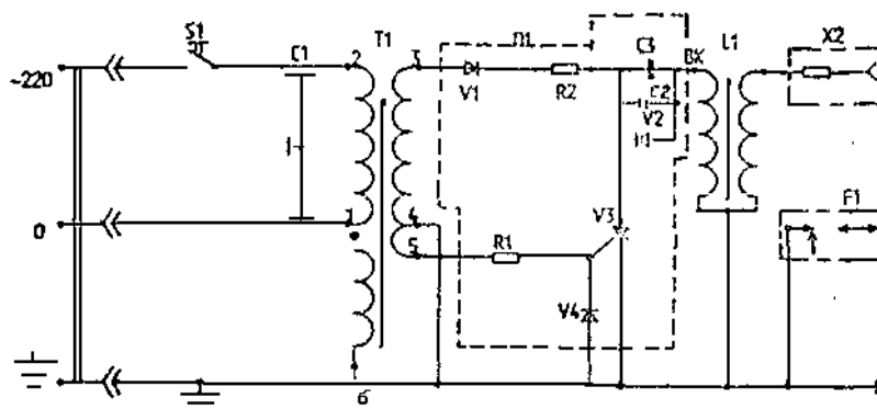
Схема электрическая принципиальная прибора Э203
