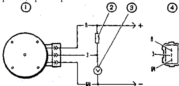
Рис. 7. Схема для проверки бесконтактного датчика на снятом датчике-распределителе зажигания: 1 - датчик-распределитель зажигания; 2 - резистор 2 кОм; 3 - вольтметр с пределом шкалы не менее 15 В и внутренним сопротивлением не менее 100 кОм; 4 - вид на штепсельный разъем датчика-распределителя зажигания
