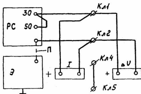
Рис.7. Схема включения реле стартера при проверке на срабатывание
