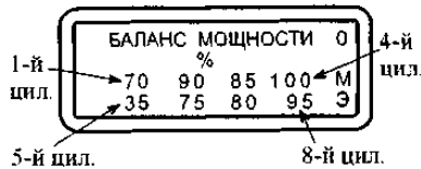
Рис.6. Порядок отображения результатов для отдельных цилиндров на примере результата теста "Баланс мощности" для 8-ми цилиндрового двигателя
