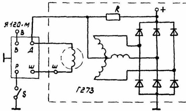
Рис.7. Схема генератора с питанием обмотки возбуждения от нулевой точки: К – сопротивление подпитки; 5 – переключатель сезонной регулировки; В – к выводу «+» аккумуляторной батареи через выключатель зажигания
