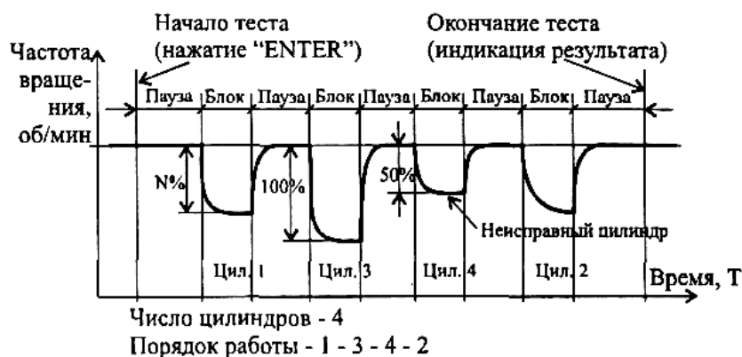
Рис.15. Баланс мощности четырехцилиндрового двигателя
