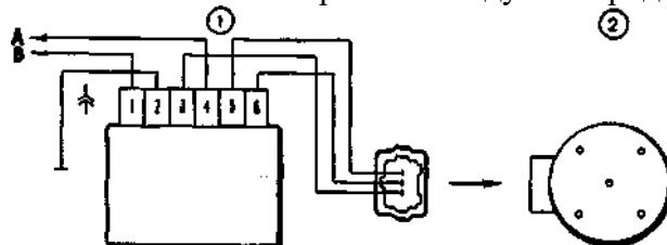
Рис. 4. Схема для снятия характеристик датчика-распределителя зажигания на стенде: 1 - коммутатор; 2 - датчик-распределитель зажигания; А - к клемме "+" стенда; В - к клемме "прерыватель" стенда
