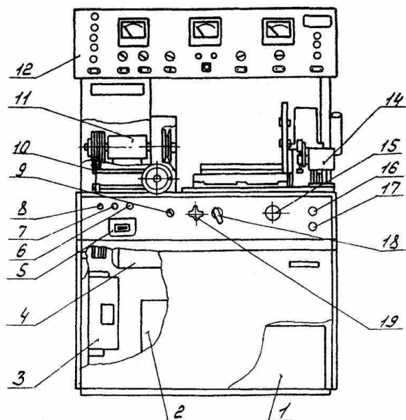
Рис.1. Стенд контрольно-испытательный
