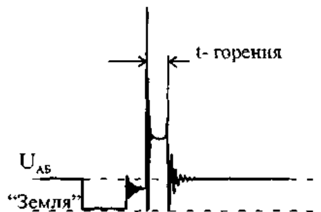
Рис.29. t-горения
