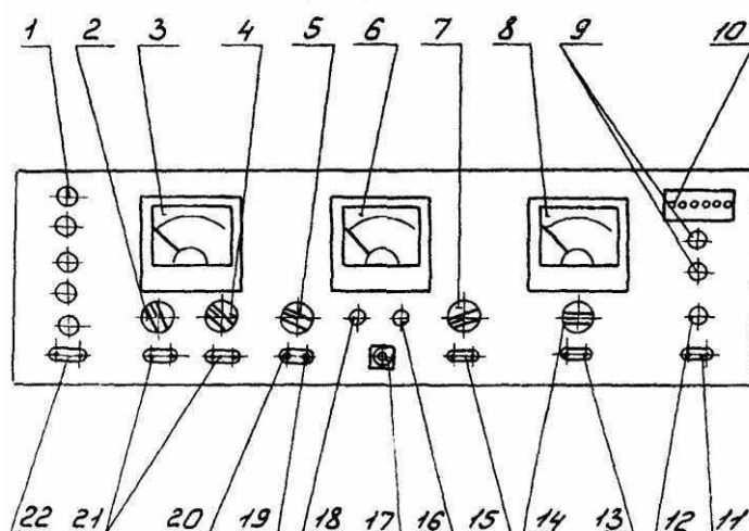
Рис.2. Панель приборов
