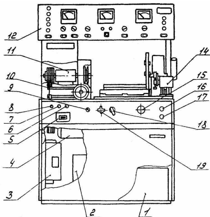
Рис.1. Стенд контрольно-испытательный
