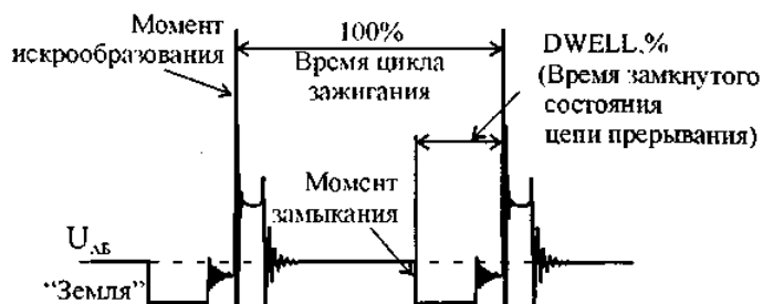
Рис.26. DWELL
