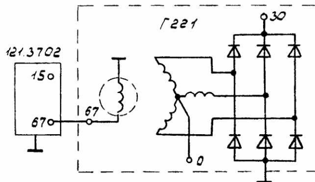
Рис.5. Схема генератора с обмоткой возбуждения, соединенной одним выводом с корпусом генератора: 15 – к «+» бортовой сети через выключатель зажигания; 67 – к потребителям; 0 – к выводу реле контрольной лампы
