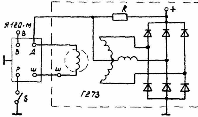
Рис.7. Схема генератора с питанием обмотки возбуждения от нулевой точки: К – сопротивление подпитки; S – переключатель сезонной регулировки; В – к выводу «+» аккумуляторной батареи через выключатель зажигания
