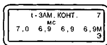
Рис.28. Тест «t-замыкания контактов»
