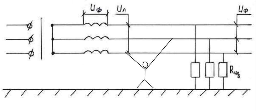
Рисунок 4. Двухфазное прикосновение
