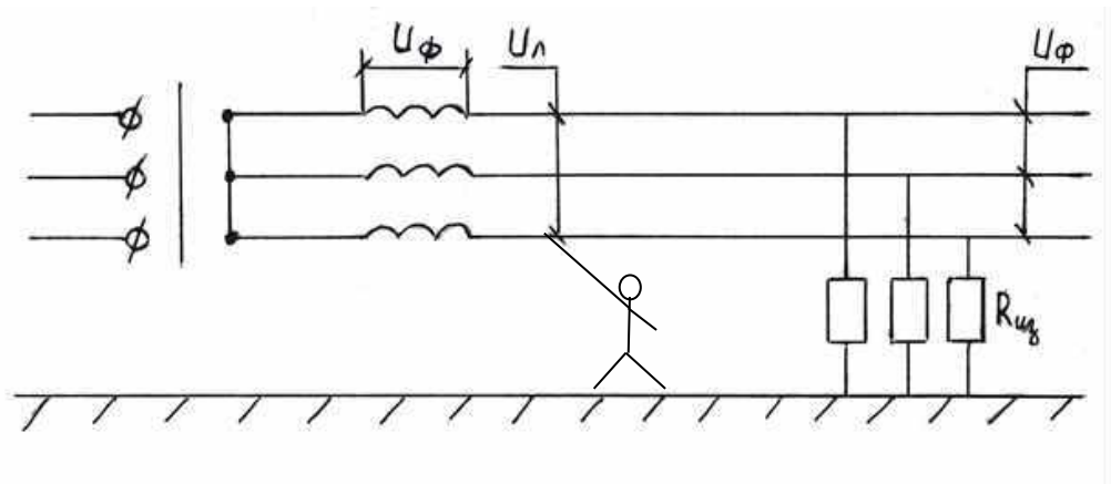
Рисунок 3. Однофазное прикосновение
