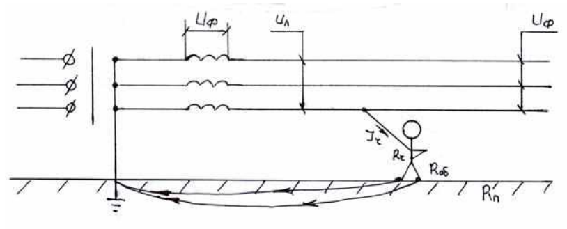
Рисунок 1. Однофазное прикосновение
