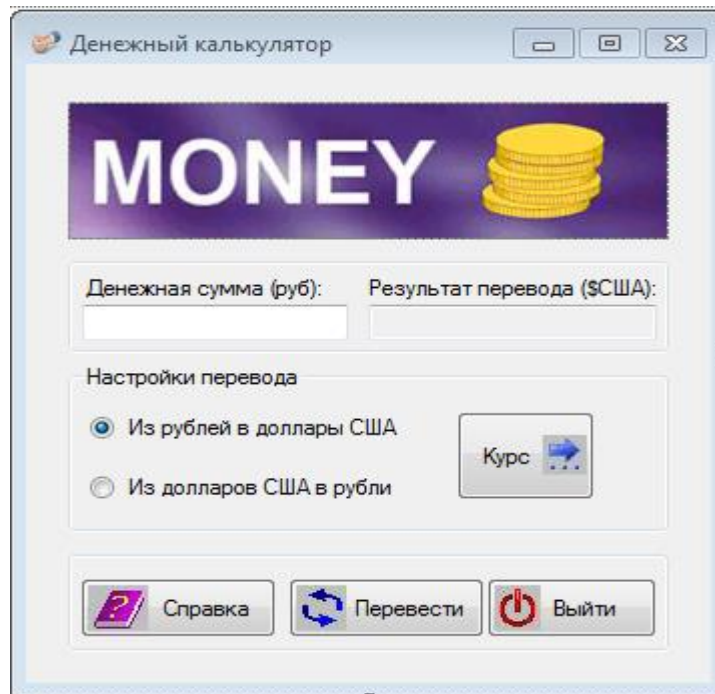
Рисунок 1 – Интерфейс приложения
