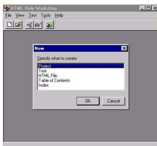
Рисунок 1- Начальный шаг
