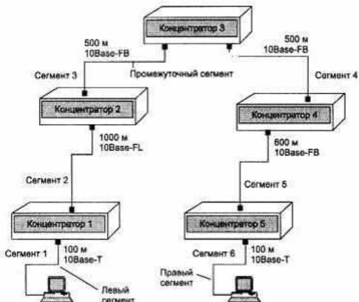
Рис. 1. Пример сети Ethernet, состоящей из сегментов различных физических стандартов
