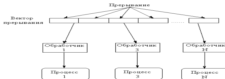
Рис. 5. Модель, управляемая прерываниями
