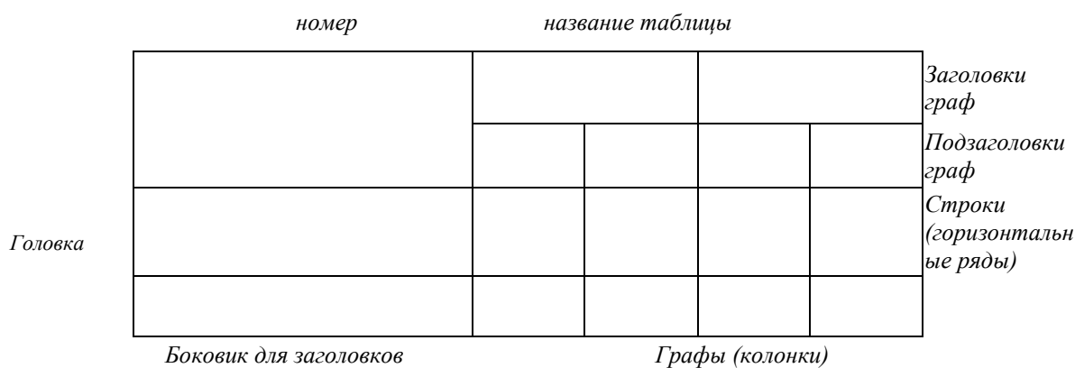
Рисунок 1 – Построение таблиц
