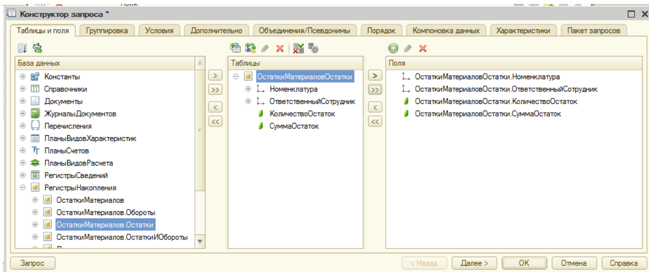
Рисунок 13.2- Создание запроса
