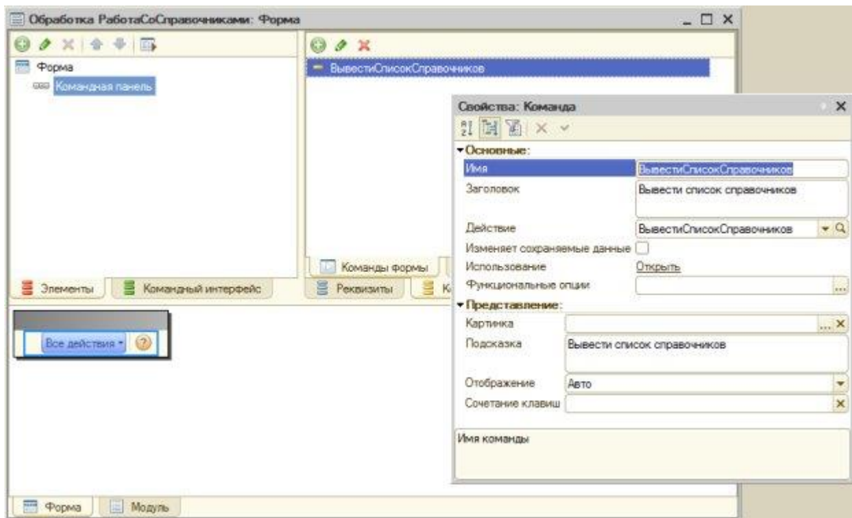
Рисунок 8.4- Настройка команды
