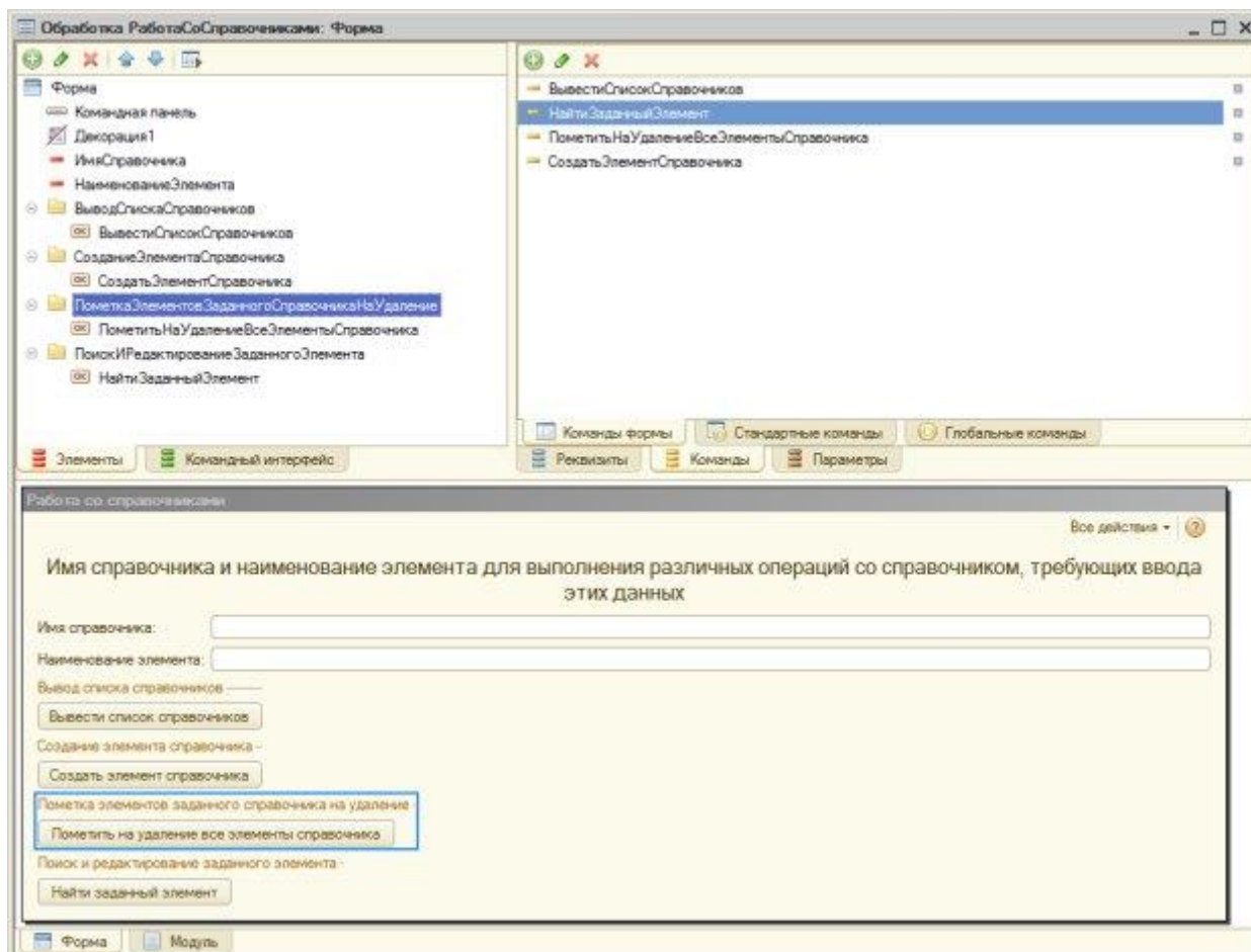
Рисунок 8.11- Переработанная форма
